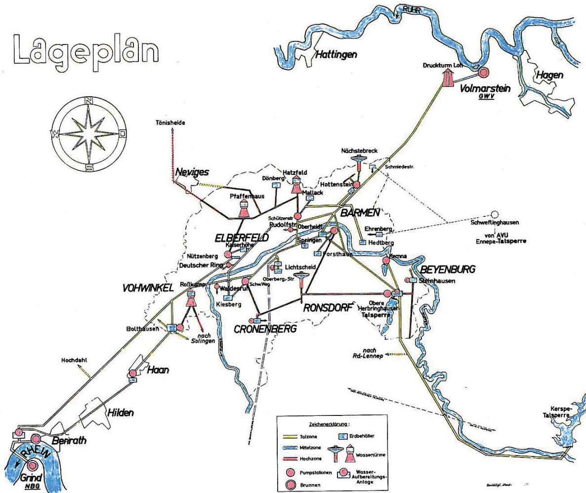
Abb. 3: Lageplan Wasserversorgung Wuppertal
